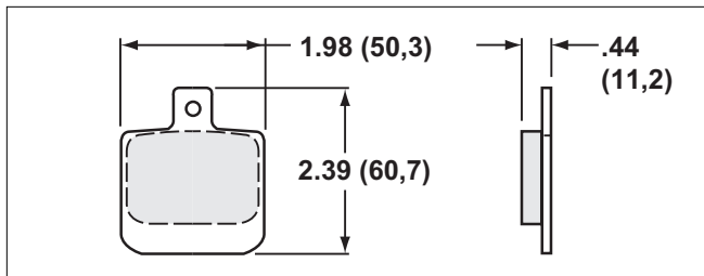
P/N 150-8272K • Dynalite Single
