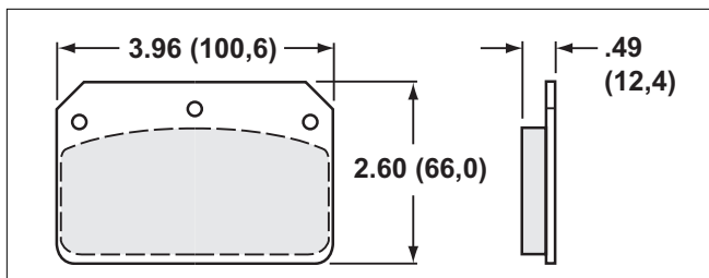
P/N 150-8450K • Dynalite
